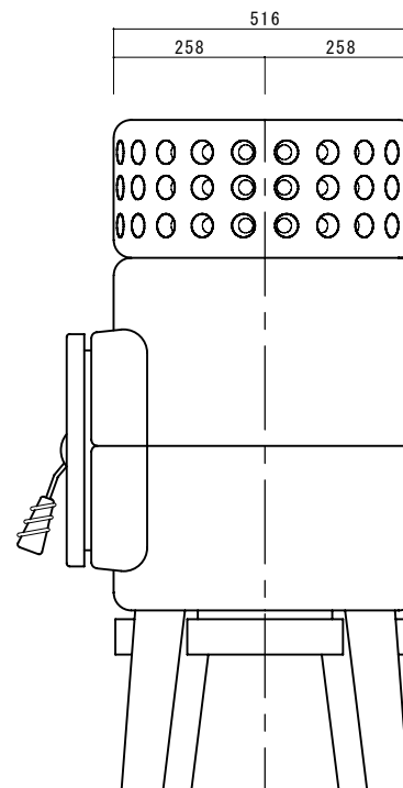
側面図
