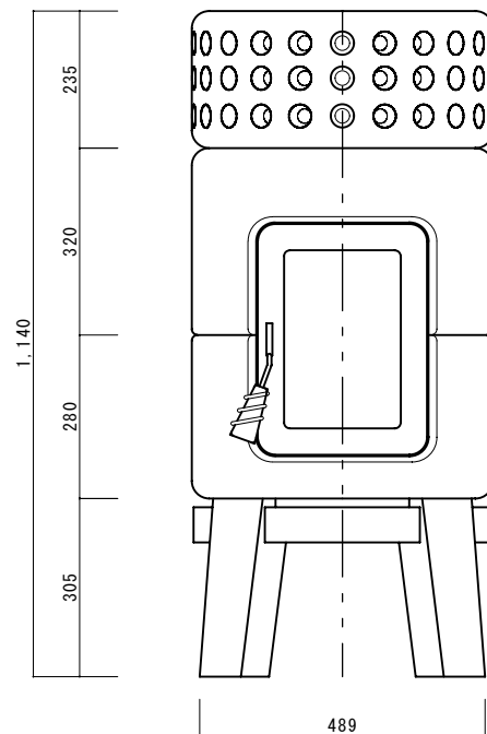
正面図
