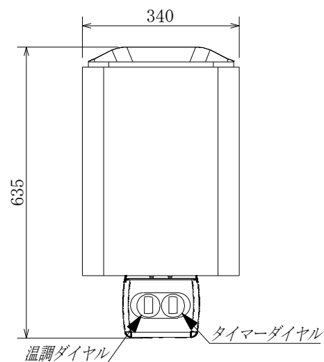
正面図
